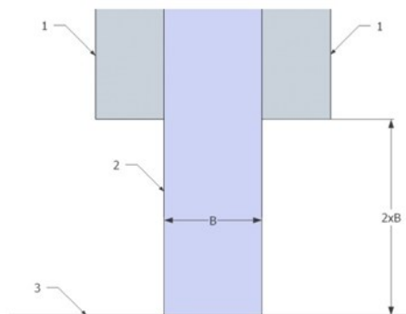
Рис. 1 Правильный монтаж очистителя 1. Крепление; 2. Резиновый скребок-очиститель серии А; 3. Поверхность ленты
