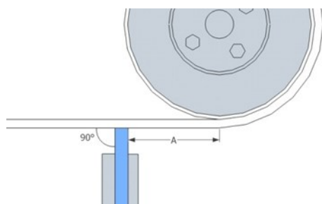
Рис. 8 Правильный монтаж скребкового очистителя. А = 50 – 80 мм
