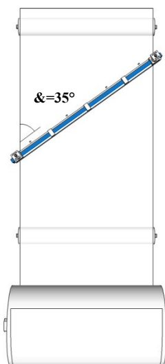
Рис. 6 Правильный монтаж диагонального очистителя. Вариант установки перед барабаном. Очиститель устанавливается исключительно на ленте между роликми холостой ветви.
