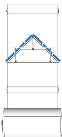
Рис. 3 Правильный монтаж плужгового очистителя. Вариант установки перед барабаном. Очиститель устанавливается исключительно на ленте между роликами холостой ветви.
