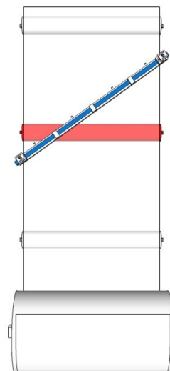
Рис. 7 Неправильный монтаж диагонального очистителя. Вариант установки перед барабаном.
