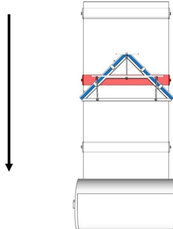
Рис. 4 Неправильный монтаж плужгового очистителя. Вариант установки перед барабаном.
