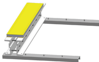
02. На направляющие швеллеры установить балку теплоизоляцией вверх.
