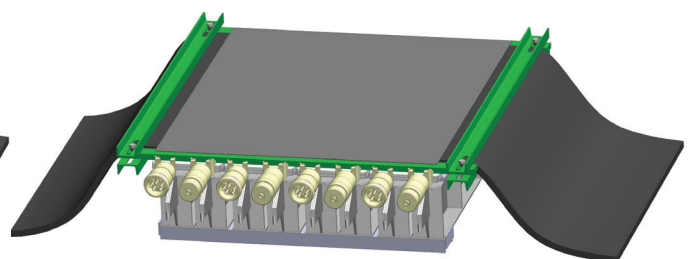
10. Собранный стык накрыть выравнивающими листами, гнездами под термометры вверх. Для предотвращения приваривания резины к металлу используется прокладочный материал.
